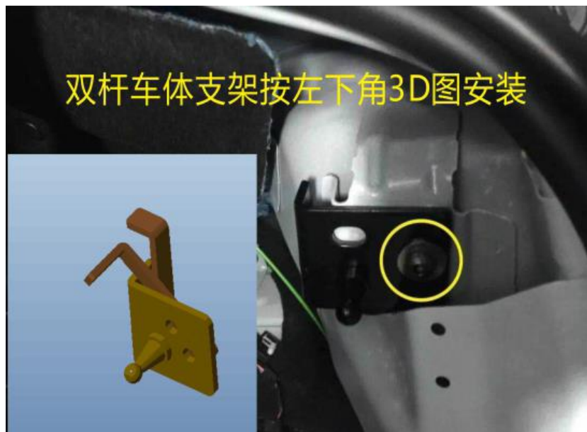
3. Установите кронштейн с шаровым наконечником и закрепите как на рисунке
