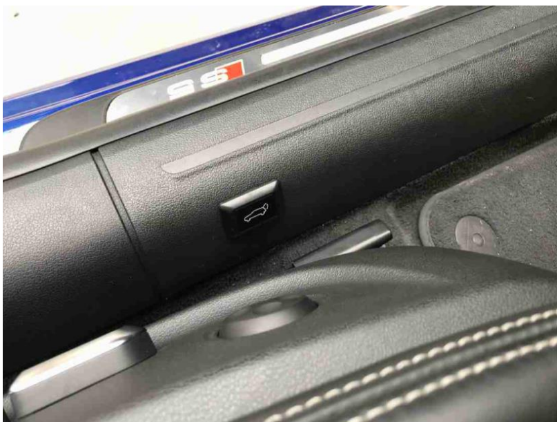
1. Рекомендуемое место установки управления приводом открывания багажника на пороге
