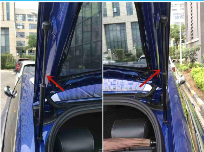
1. Снимите штатные стойки
